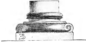
Fig. 61. Ionic Base.
